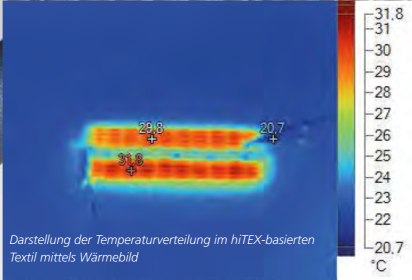
Gewebtes Heizband mit hiTEX
